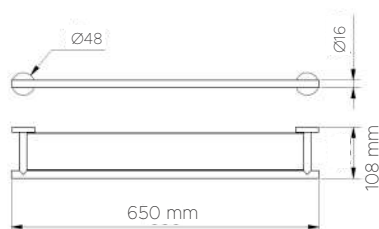
DATOS TÉCNICOS DATI TECNICI 05151
