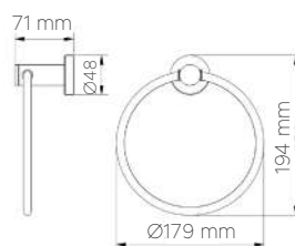
DATOS TÉCNICOS DATI TECNICI 05152
