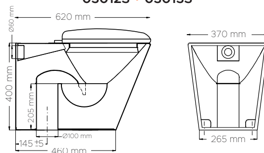
DATOS TÉCNICOS DATI TECNICI 03012S • 03013S
