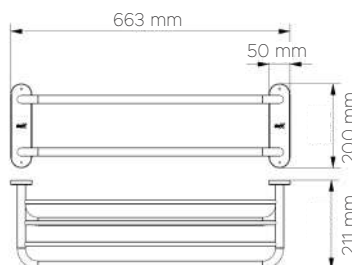
DATOS TÉCNICOS DATI TECNICI 05003
