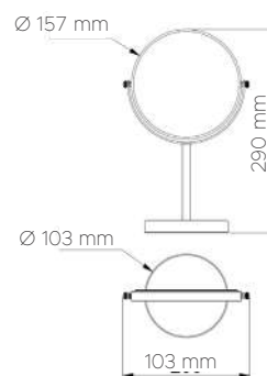
DATOS TÉCNICOS DATI TECNICI 05197
