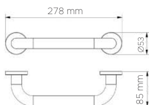
DATOS TÉCNICOS DATI TECNICI 05150
