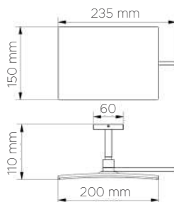
DATOS TÉCNICOS DATI TECNICI 05164
