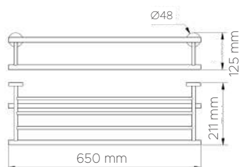
DATOS TÉCNICOS DATI TECNICI 05156
