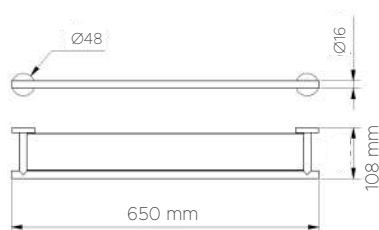
DATOS TÉCNICOS DATI TECNICI 05149
